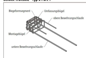
Schöck Tronsole® Typ Z Part T
